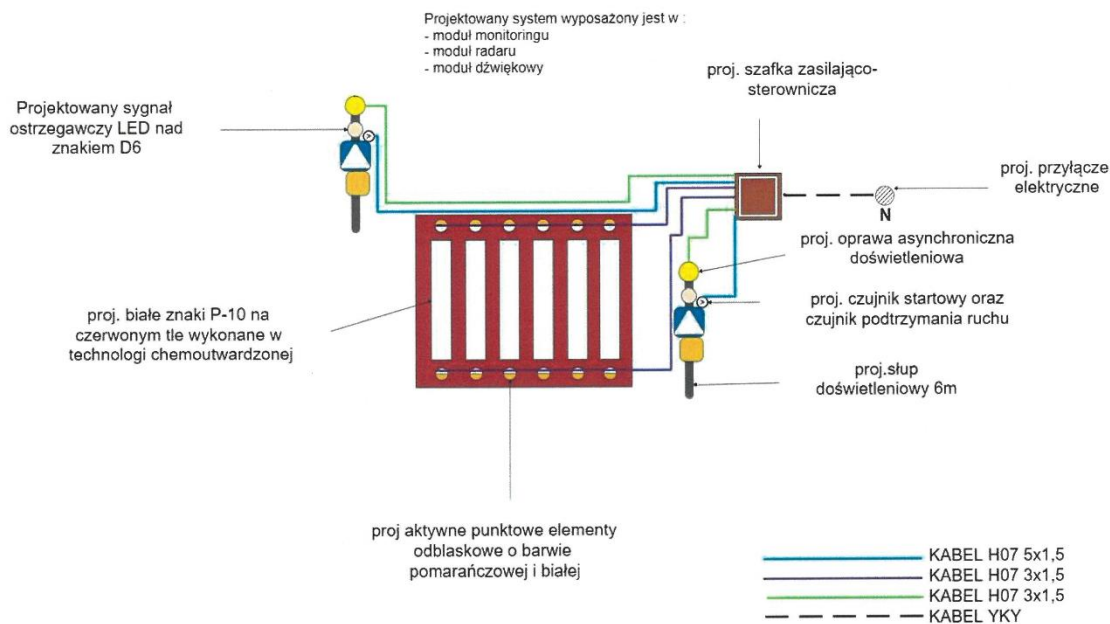
Rys. 1 Przykładowy schemat przejścia dla pieszych
