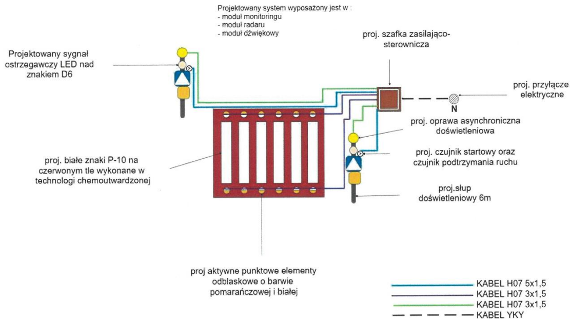
Rys. 1 Przykładowy schemat przejścia dla pieszych
