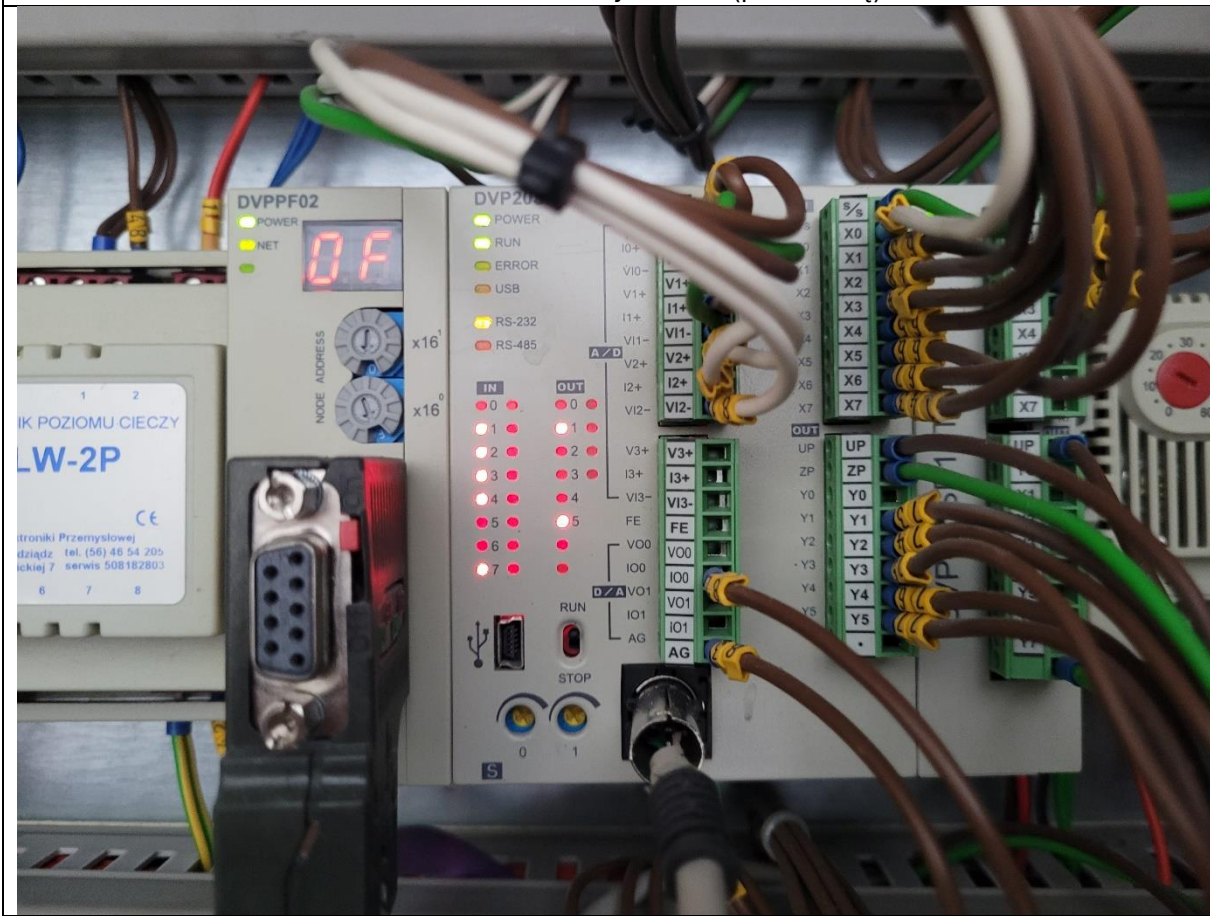
Szafa S5 - Sterownik Hydroforni (poza szafą)
