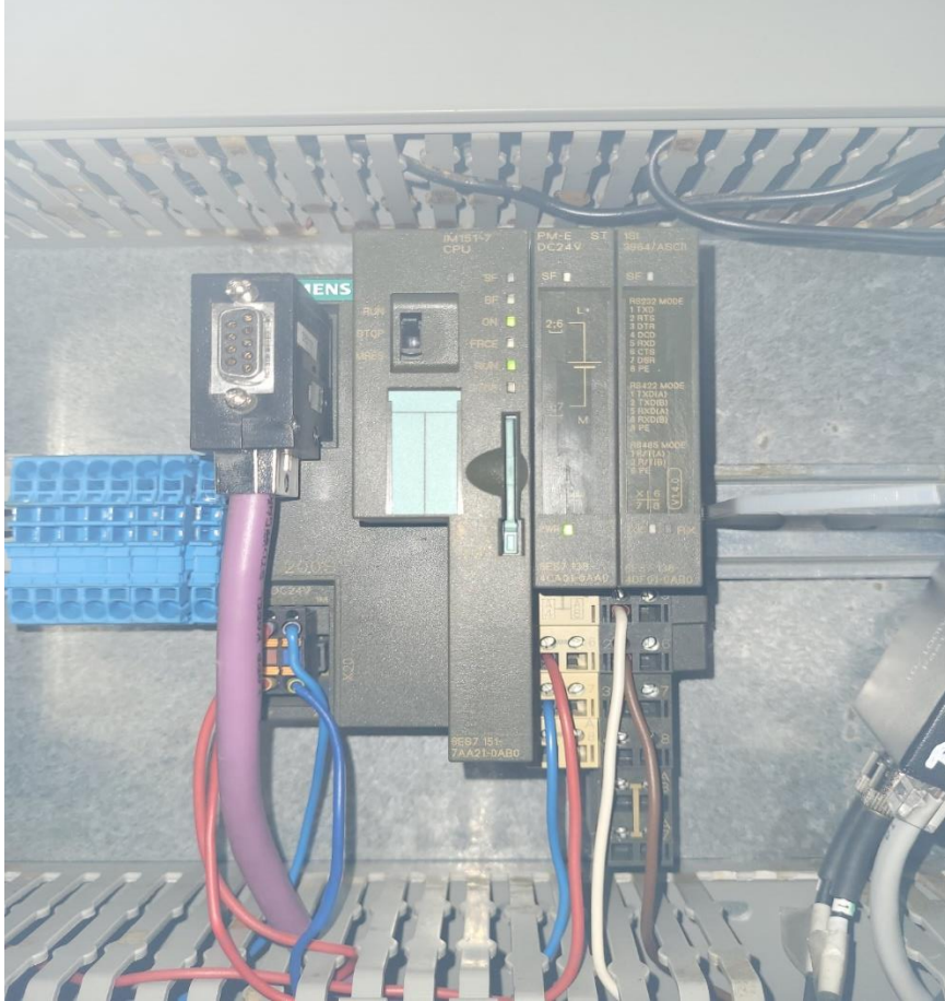
Szafa S7 – liczniki energii elektrycznej (całość przetożona do nowej szafy)
