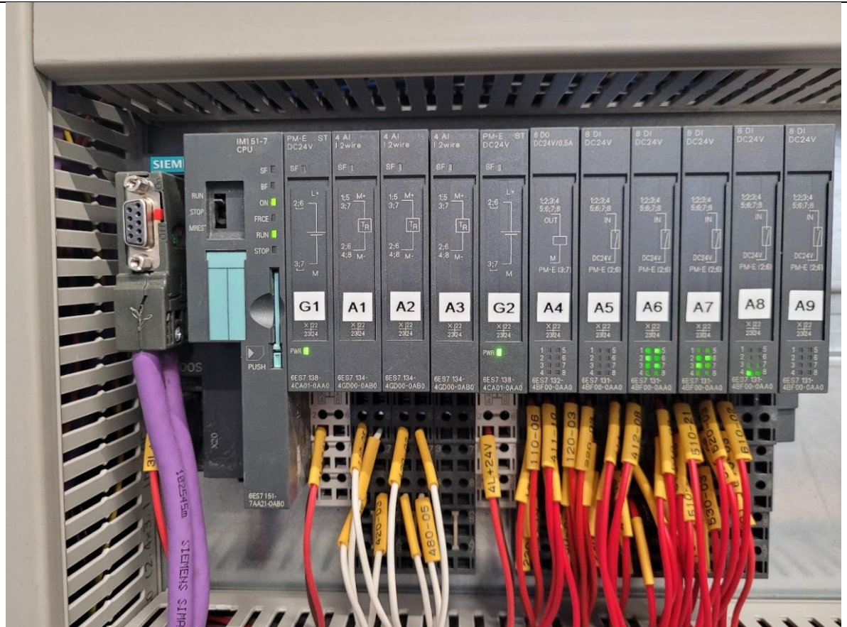
Szafa S6 – Sterownik szafy ATARA (poza szafą)
