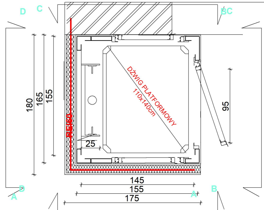
Rzut na kondygnacji 2 i 3 1:25
