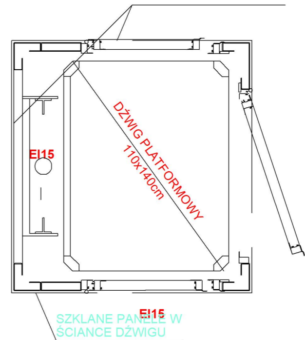
Rzut na kondygnacji 1 1:25
