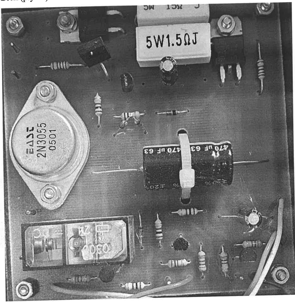
Blok (płytki) sterowania WSB03
