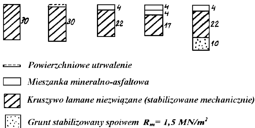
Rys. 4. Przykładowe wybrane konstrukcje nawierzchni utwardzonego pobocza z kruszywami łamanymi niezwiązanymi
