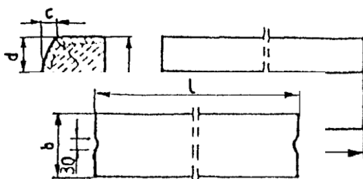
Rys. 1. Wymiarowanie krawężników
