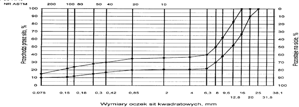
Rys. 2. Krzywe graniczne uziarnienia mieszanki mineralnej BA od 0 do 20 mm (mieszanka o nieciąglym uziarnieniu) do warstwy ścieralnej nawierzchni drogi o obciążeniu ruchem od KR3 do KR6
