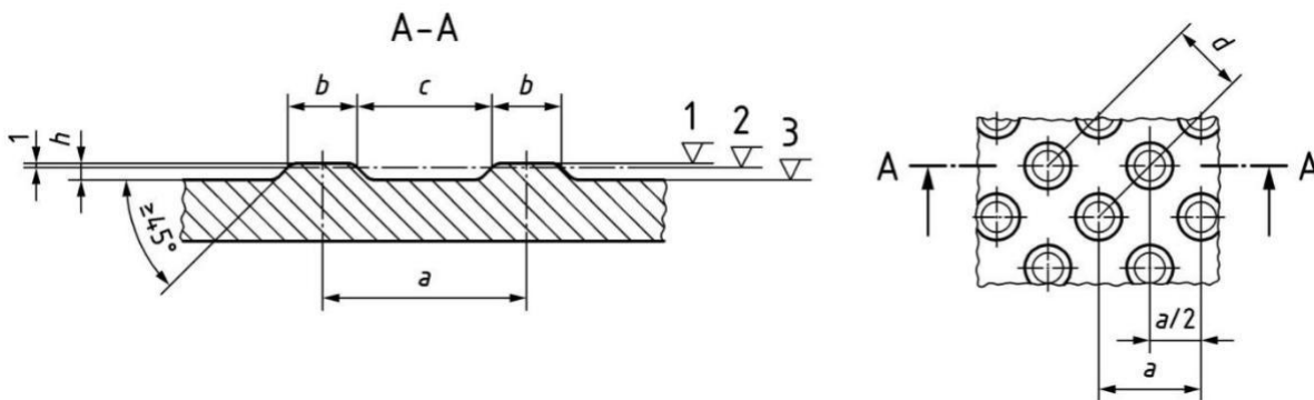
Rys 1. Wymiary wypustek płytki ostrzegawczej na podstawie normy DIN 32984.
