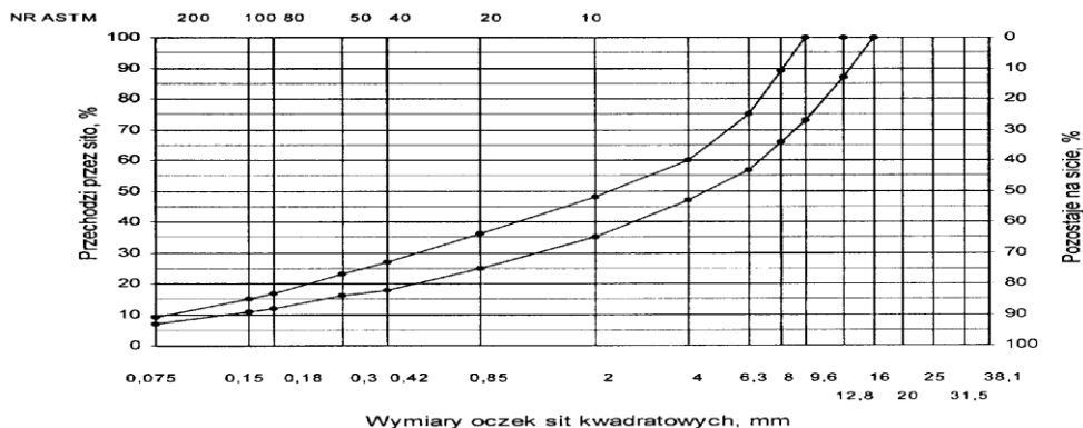
Rys. 4. Krzywe graniczne uziarnienia mieszanki mineralnej BA od 0 do 12,8 mm do warstwy ścieralnej nawierzchni drogi o obciążeniu ruchem od KR3 do KR6
