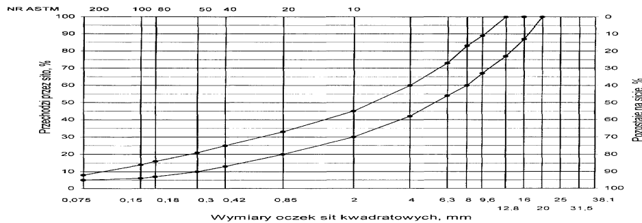
Rys. 5. Krzywe graniczne uziarnienia mieszanki mineralnej BA od 0 do 20 mm do warstwy wiążącej, wyrównawczej i wzmacniającej nawierzchni drogi o obciążeniu ruchem od KR3 do KR6
