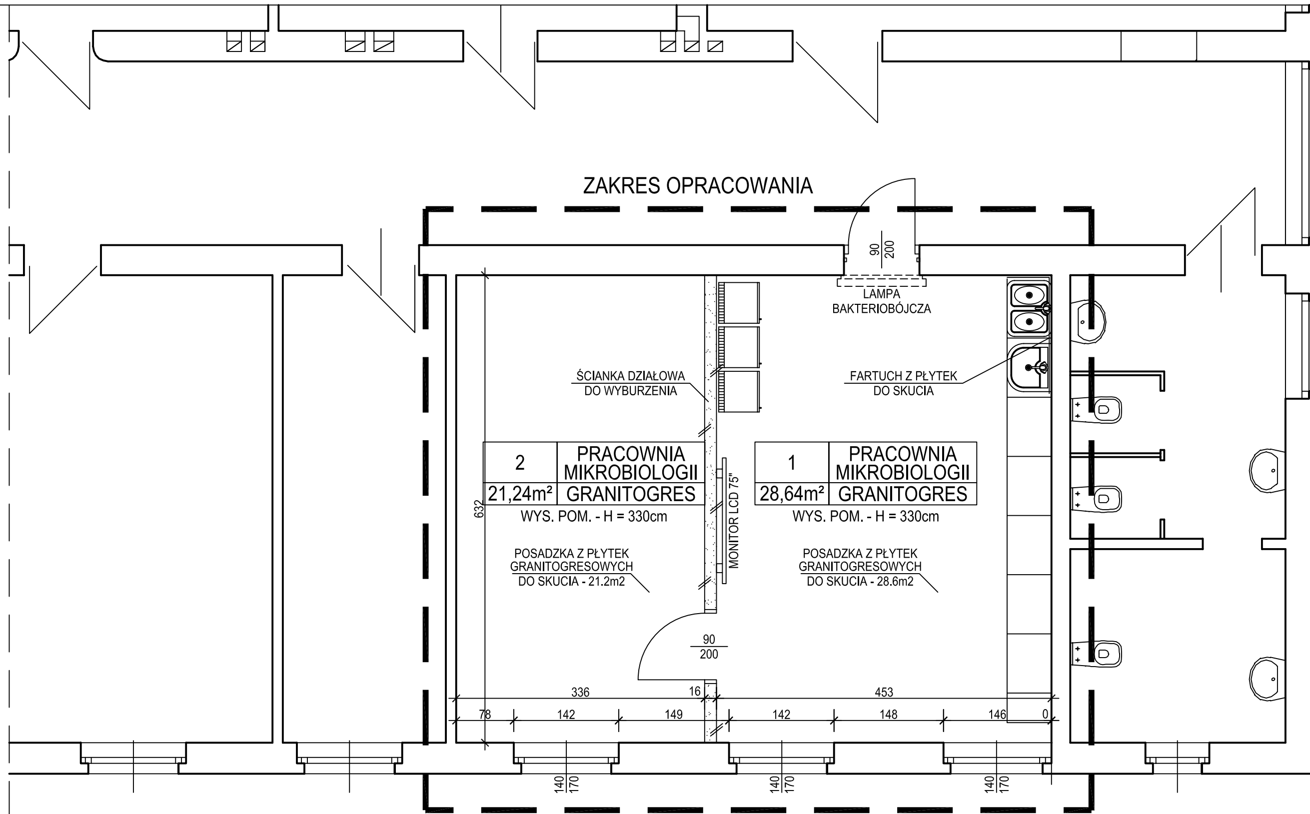
RZUT II PIĘTRA PRACOWNIA BICHEMII I MIKROBIOLOGII - INWENTARYZACJA I ROZBIÓRKI
