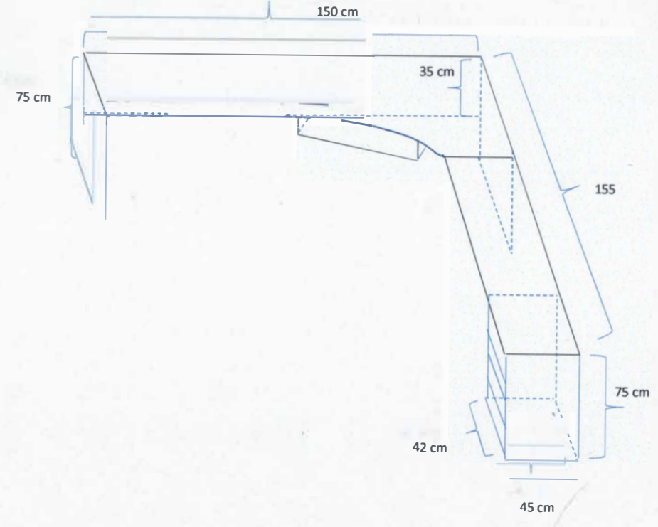
Biurko narożne z szufladami i szufladą na klawiaturę – widok z przodu
