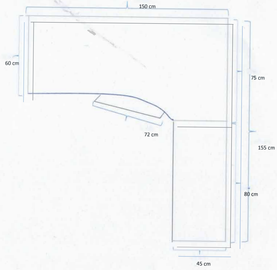
Biurko narożne – widok z góry
