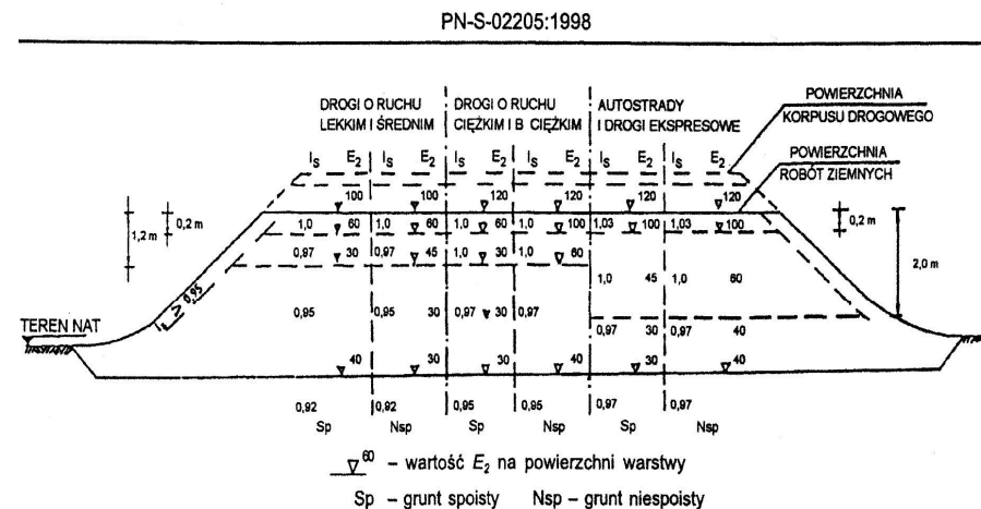
Rysunek 3 - Wartości wymagane w nasypach: wskaźnika zagęszczenia I_e i wtórnego modułu odkształcenia E_2 , megapaskali
