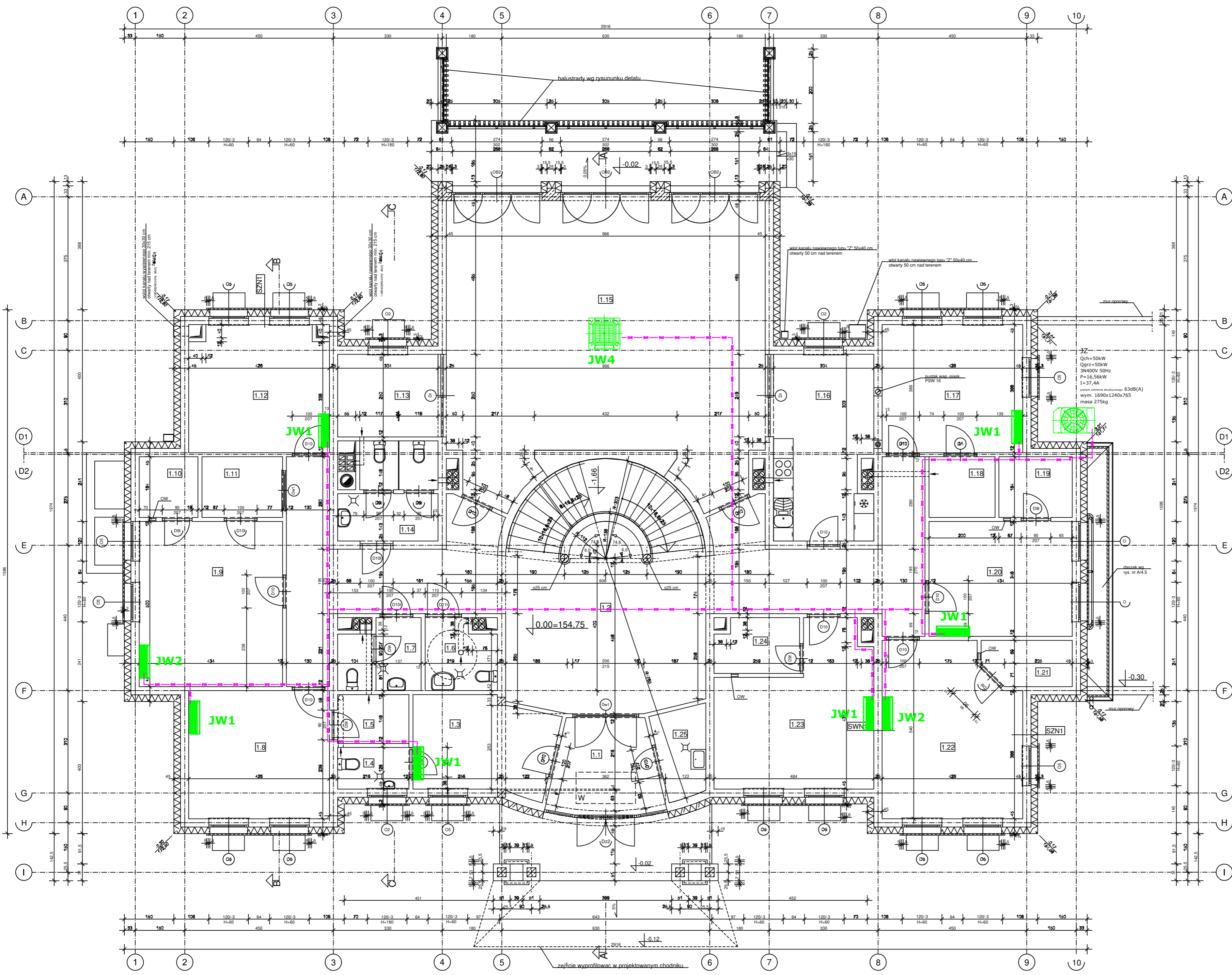
RZUT PARTERU
