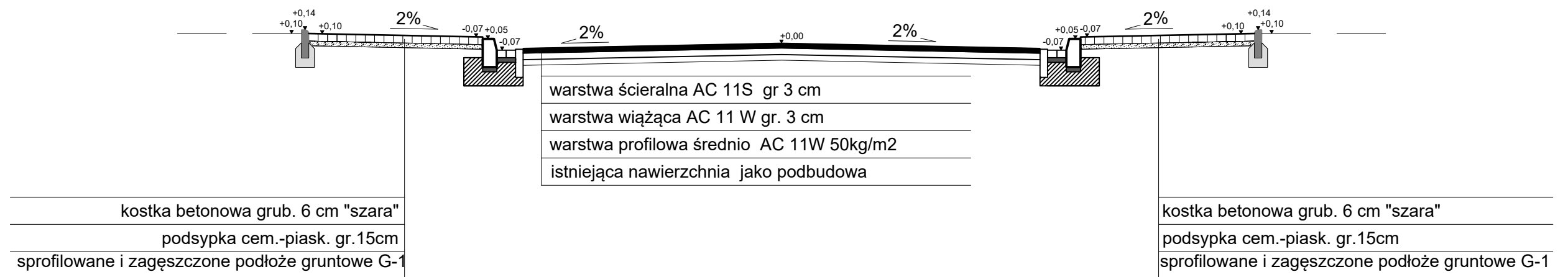
Szczegół B
