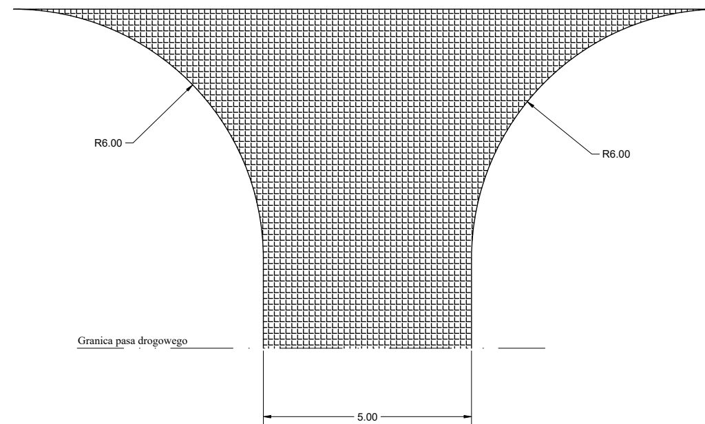
Przekrój zjazd
