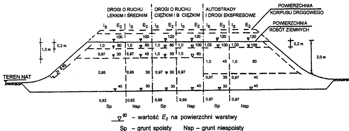
Rysunek 3 – Wartości wymagane w nasypach: wskaźnika zagęszczenia I_s i wtórnego modułu odkształcenia E_2 , megapaskall
