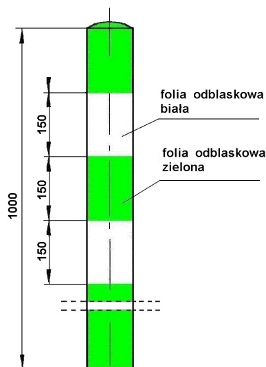
Rys. 3. Słupek krawędziowy U-2
