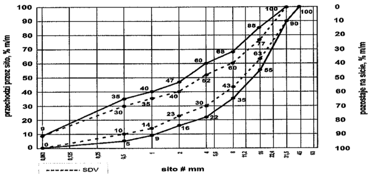
Rys. 18. Uziarnienie mieszanki niezwiązanej 0/31,5 dla podbudowy zasadniczej
