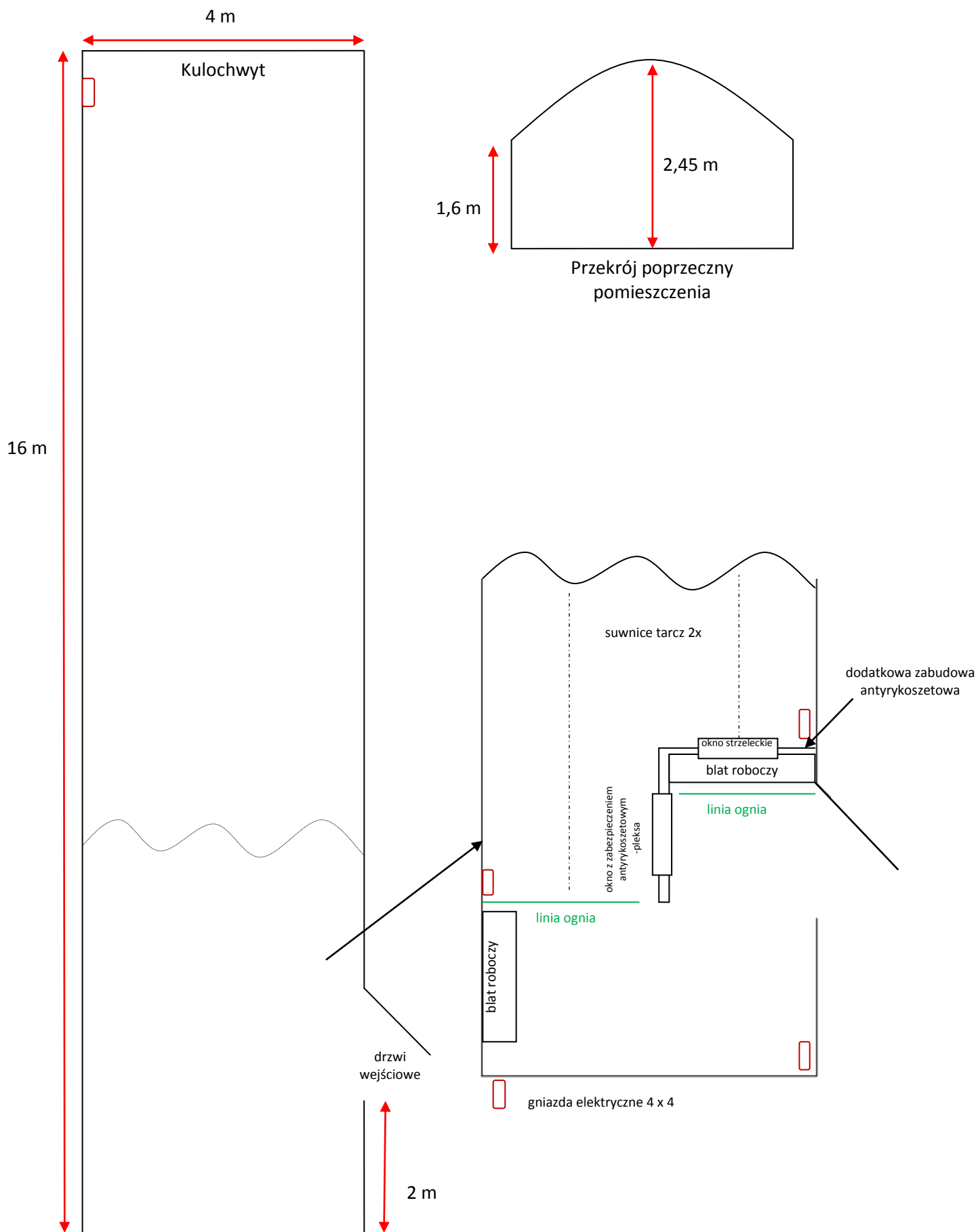
Rzut z góry Pomieszczenie przeznaczone na dwa stanowiska badawcze
