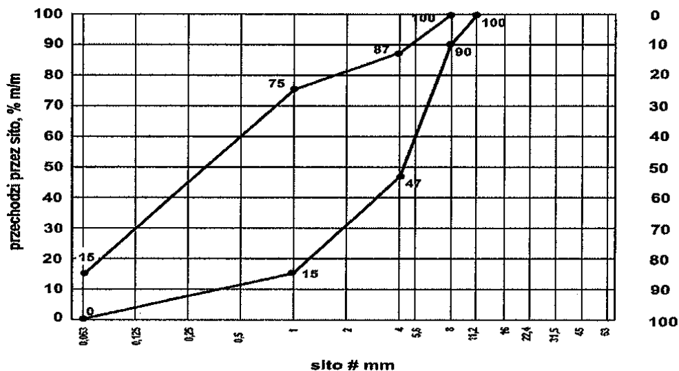
Rys. 1. Krzywe graniczne uziarnienia mieszanki kruszywo 0/8 mm do górnej warstwy podłoża ulepszonego
