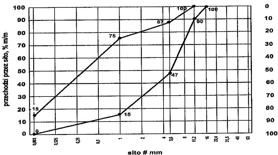
Rys. 2. Krzywe graniczne uziarnienia mieszanki kruszywo 0/11,2 mm do górnej warstwy podłoża ulepszonego
