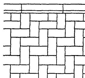
Rys. 6. Przykłady deseni układania betonowych kostek brukowych (typu Holland – wg jw.)
