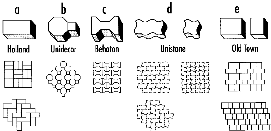
Rys. 5. Najczęściej spotykane kształty kostek i sposoby ich układania
