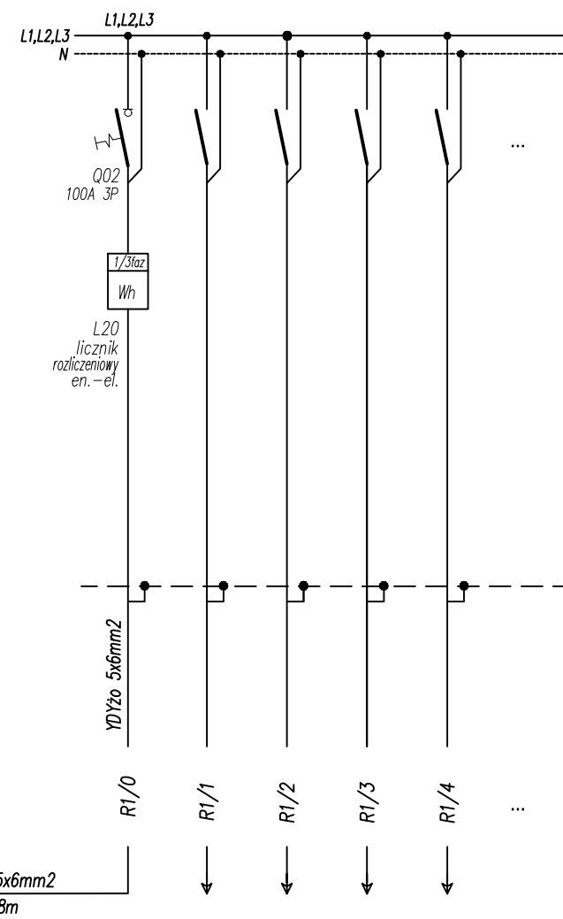
Tablica licznikowo-bezpiecznikowa 230/400V - R1
