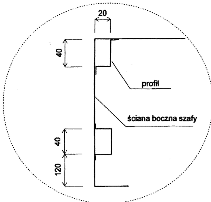
Szczegół B
