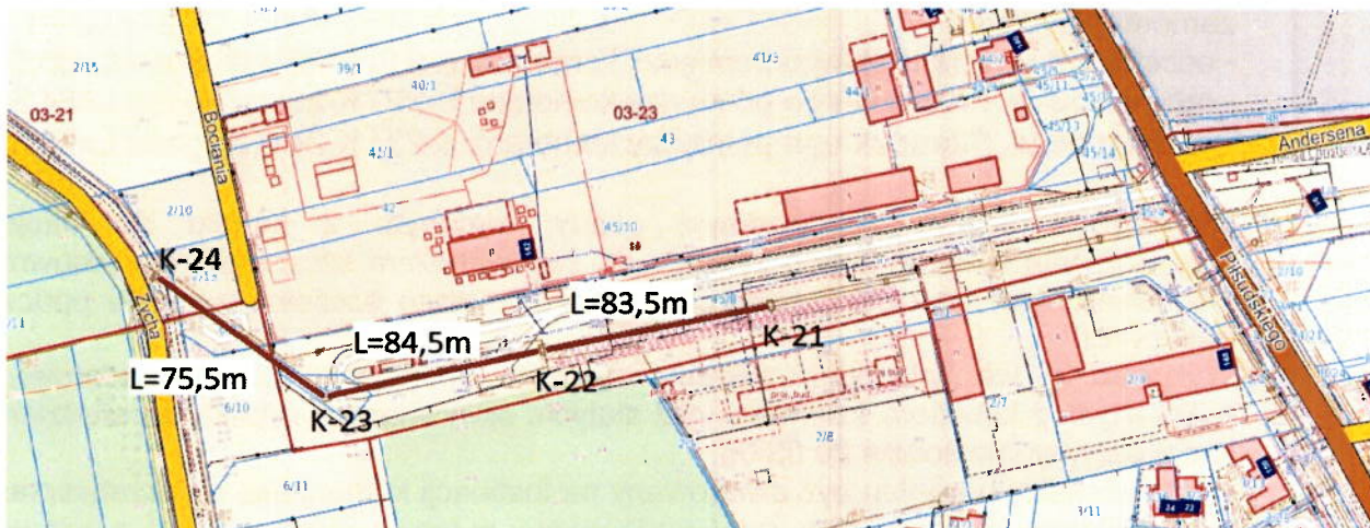
Rys.1 Kolektor ściekowy w ul. Sezamkowej w Żąbkach i Klamrowej w Warszawie.
