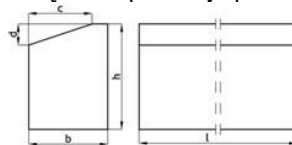
krawężnik wyspowy
