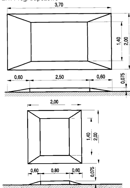
Rys. 2. Przykłady wymiarowania progów zwalniających wyspowych (wg [23])
