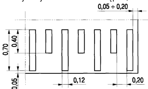
Rys. 2. Oznakowanie poziome progu zwalniającego
