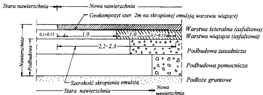
Rys. 2. Konstrukcja połączenia starej i nowej nawierzchni
