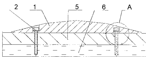
Rys. 4. Przykład umocowania progu do nawierzchni jezdni
