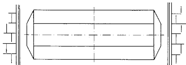
Rys. 2. Przykłady wymiarowania progów zwalniających wyspowych (wg [23])
