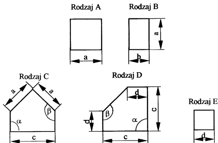
Rysunek 1. Rodzaje płyt chodnikowych betonowych Tablica 1. Wymiary płyt chodnikowych betonowych
