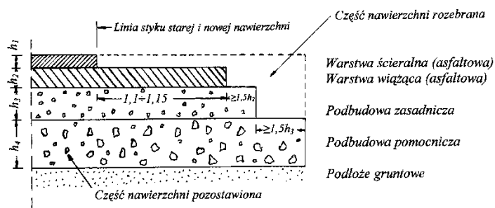
Rys. 1. Sposób rozebrania nawierzchni istniejącej
