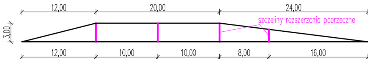
Rys.1. Schemat rozmieszczenia szczelin rozszerzenia poprzecznych
