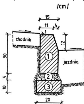
Rys. 1. Przykładowe ustawienie krawężników na łąwie betonowej
