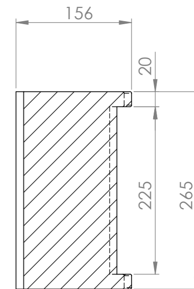
PRZEKRÓJ B-B
