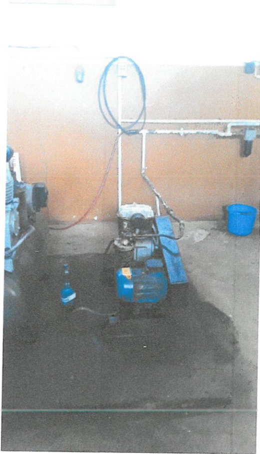
Układ przygotowania powietrza technologicznego
