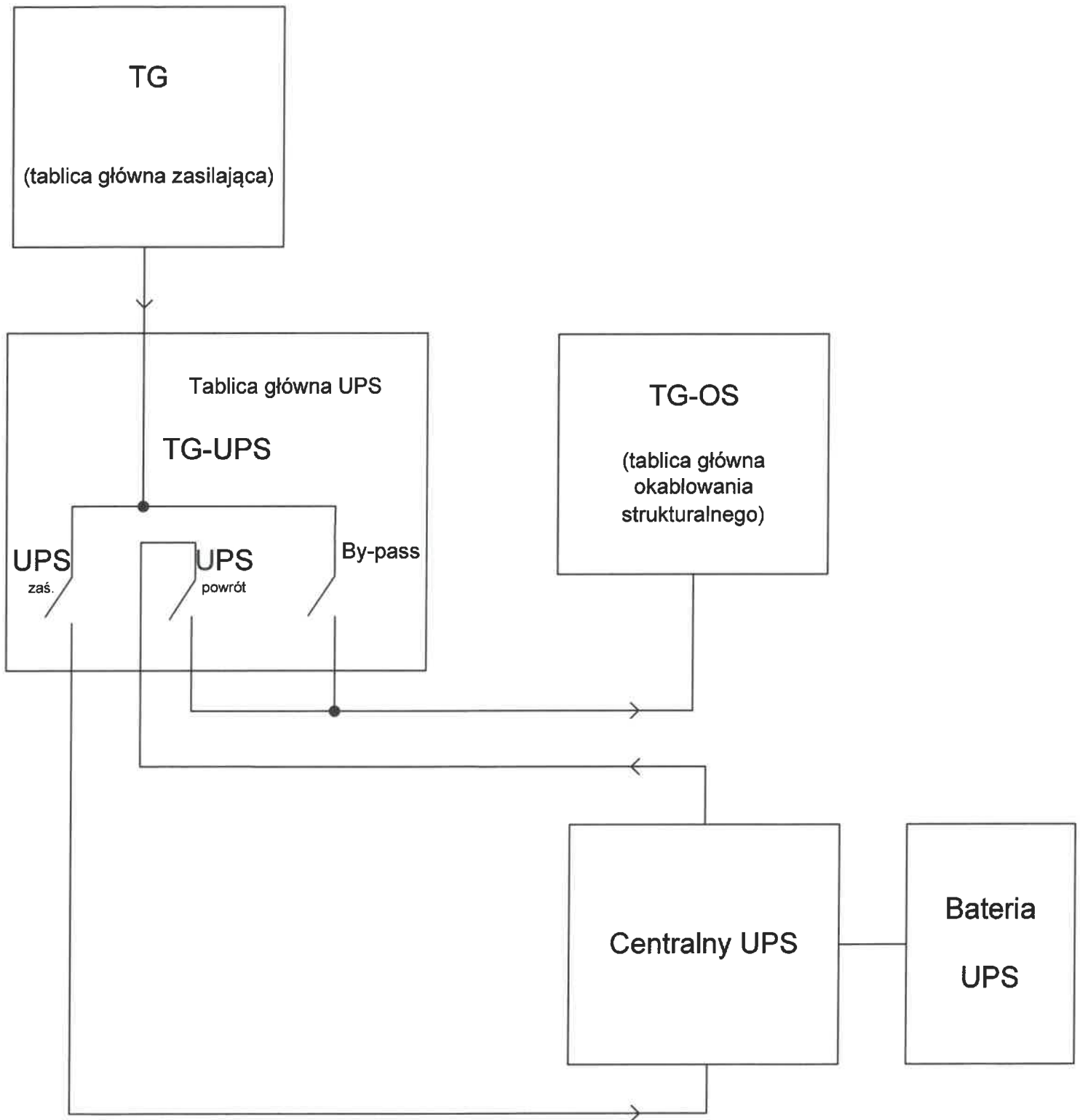
Rysunek przedstawiający koncepcję BY-PASS-u.
