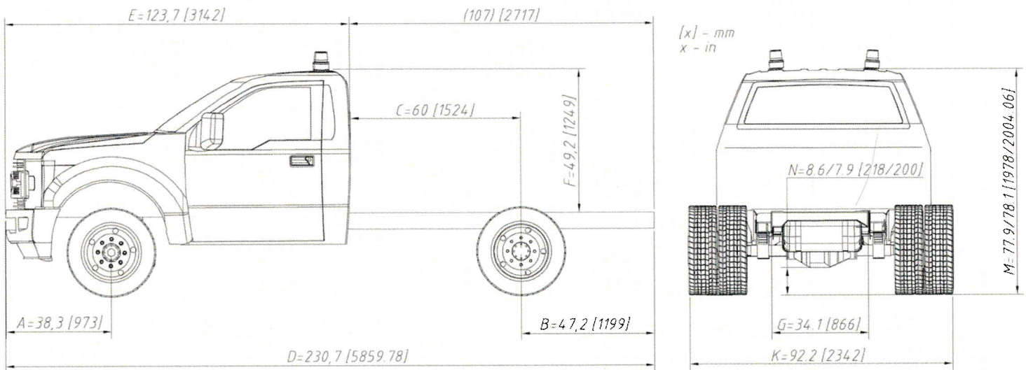
Rys. 1 Wymiary katalogowe samochodu FORD F350 Havy-Duty 145.3"
