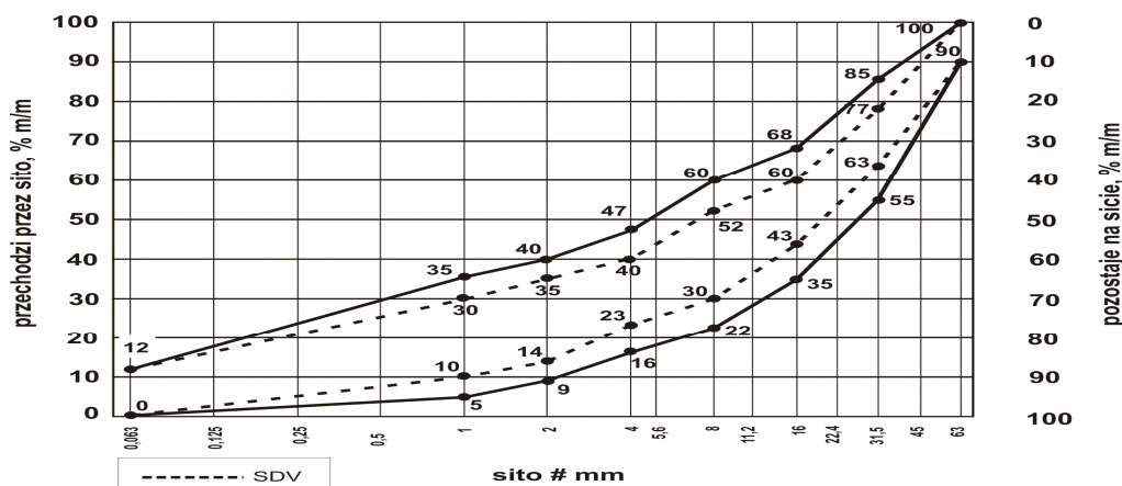
Rys. 1. Mieszanka niezwiązana 0/63 do warstwy podbudowy pomocniczej
