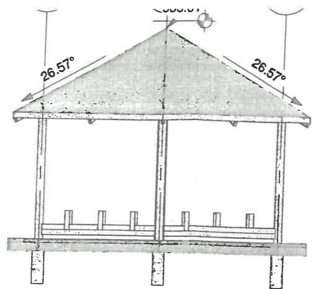
3 Wschód 1 : 100
