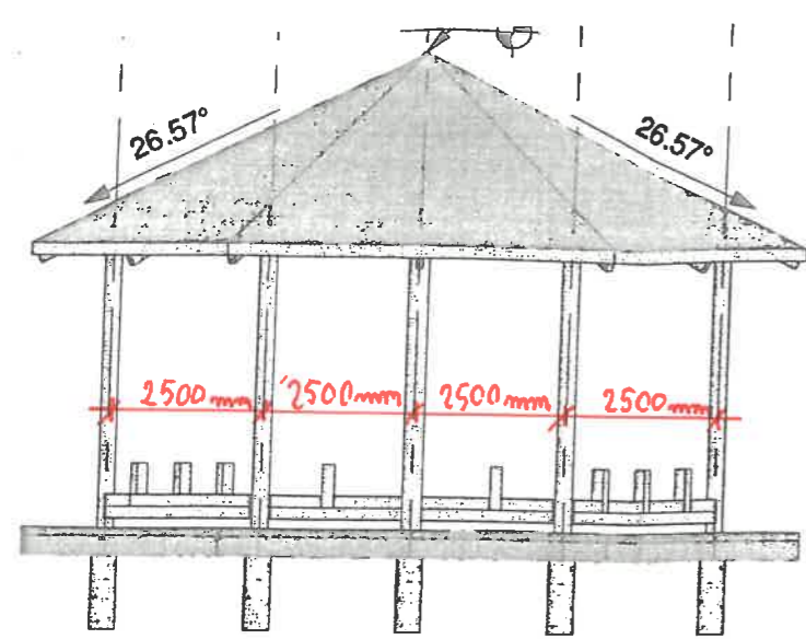
1 Południe 1 : 100
