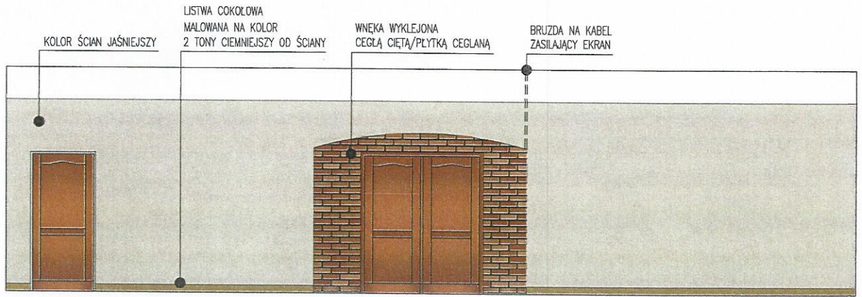
KŁAD ŚCIANY Z WEJŚCIEM DO KAWIARNI
