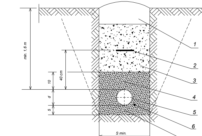
PROFIL WYKOPU DLA RUR Z PE
