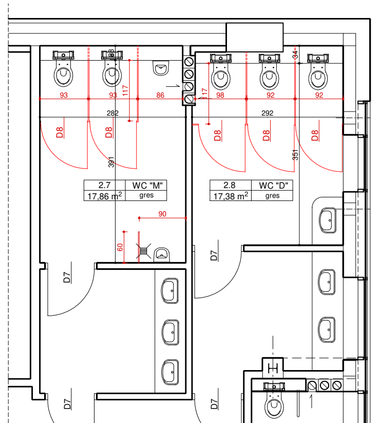
RZUT PIĘTRA
