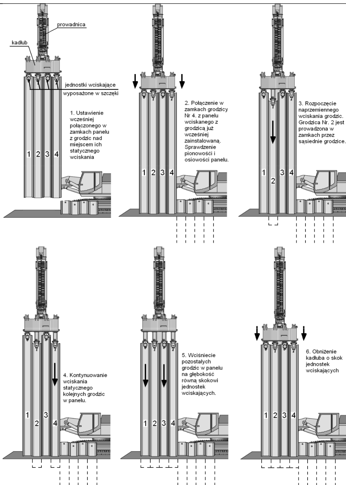
Rysunek 3. Procedura wciskania grodzic urządzeniem mocowanym do masztu prowadzącego 5.5.4. Ramy prowadzące
