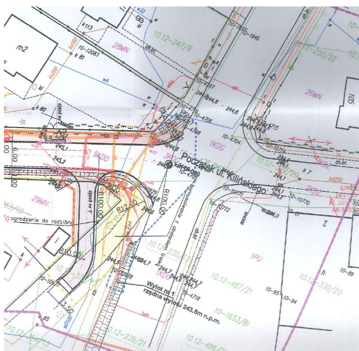
fragment planu sytuacyjnego z dokumentacji Rozbudowa i przebudowa ulicy Wyzwolenia i Kilińskiego w Jastrzębiu-Zdroju
