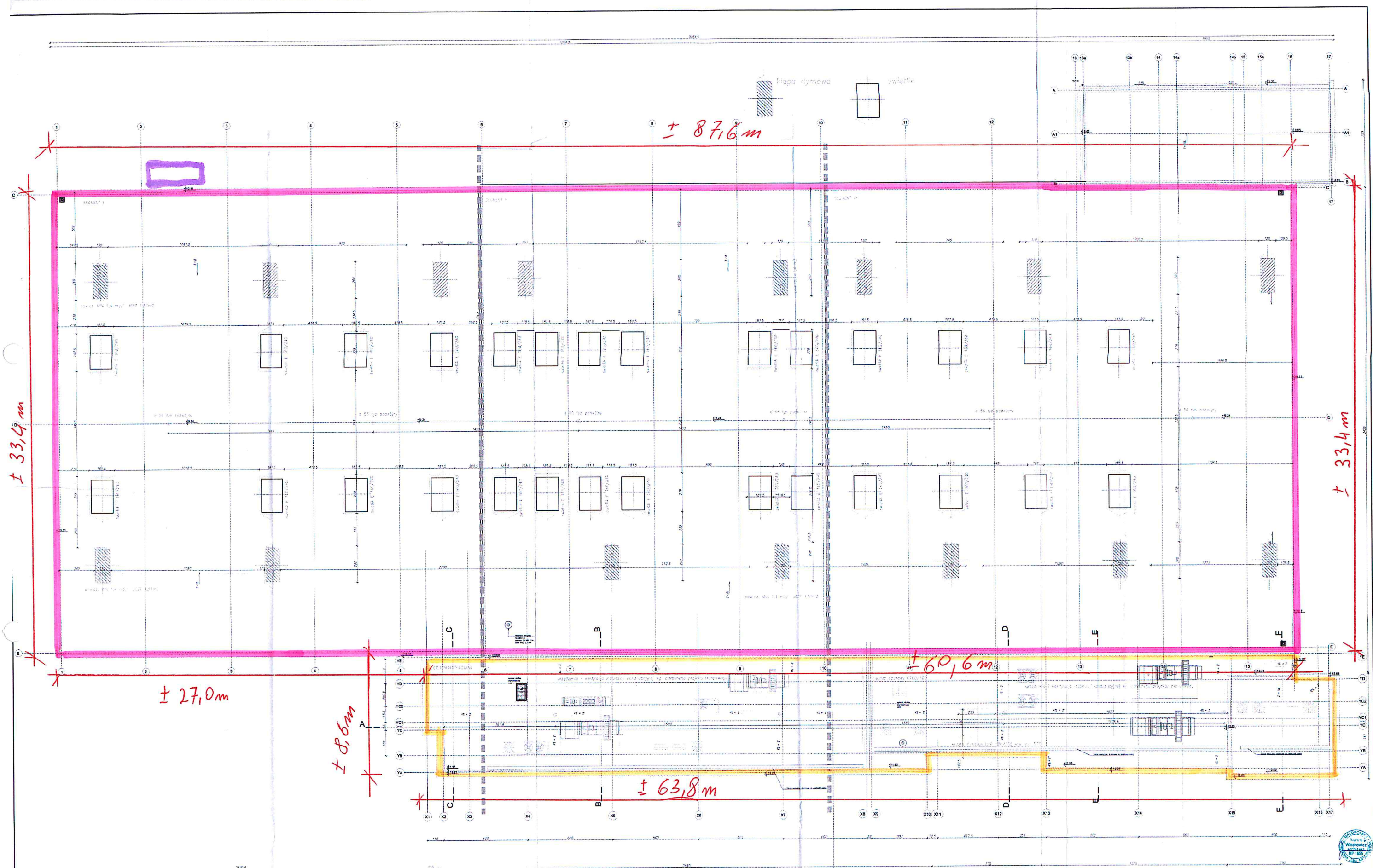
Rys Nr. 2 - Wymiary budynku (poprzecznie)
