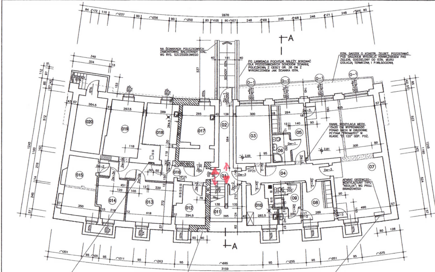
RZUT PIWNIC skala 1:100
