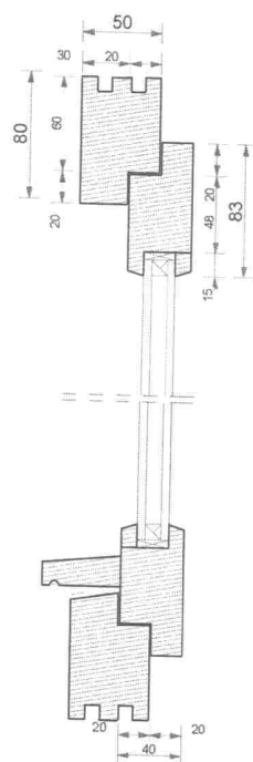
Przekrój pionowy,
