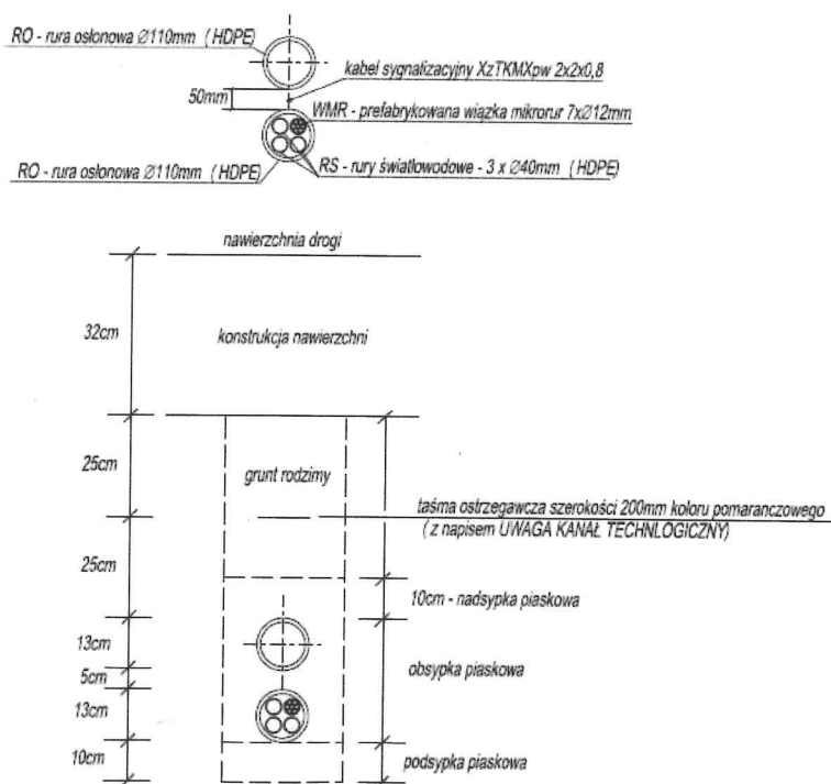
KANAŁ TECHNOLOGICZNY ULICZNY - KTp1 SKALA 1:10
