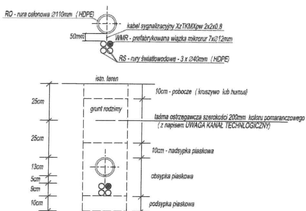
KANAŁ TECHNOLOGICZNY ULICZNY - KTu1 SKALA 1:10
