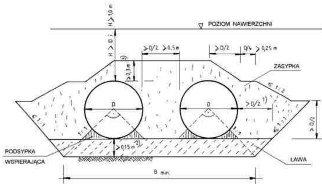
Rys. nr 2. : Zasyпка nad przepustem dwururowym
