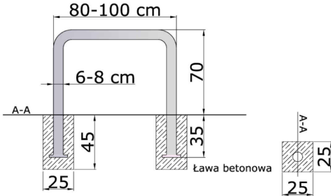
Przykładowy stojak rowerowy „odwrócone U”.
