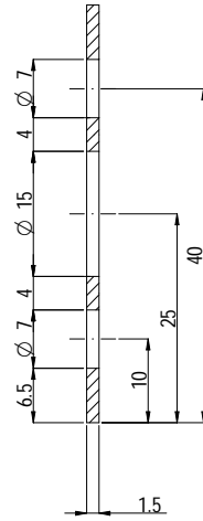
A-A SCALE 1:1
