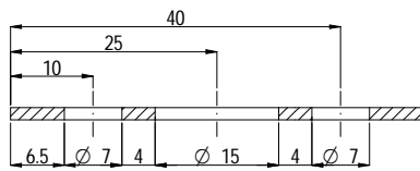
B-B SCALE 1:1
