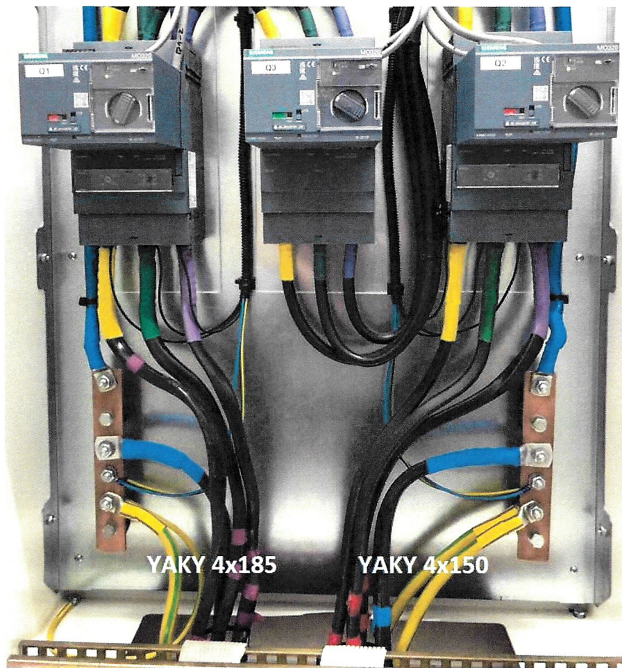
Podjęcia linii kablowych K1 na SZR rozdzielnicy R10-4.
