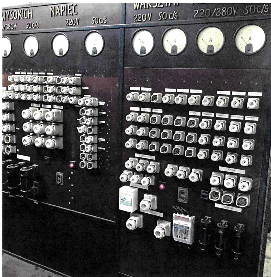
Widok rozdzielnicy RWt, front – fragment.
