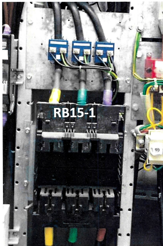
Widok zabezpieczenia RB15-1 w Polu 2 rozdzielnicy R10-4, zasilania rezerwowego R10-15.
