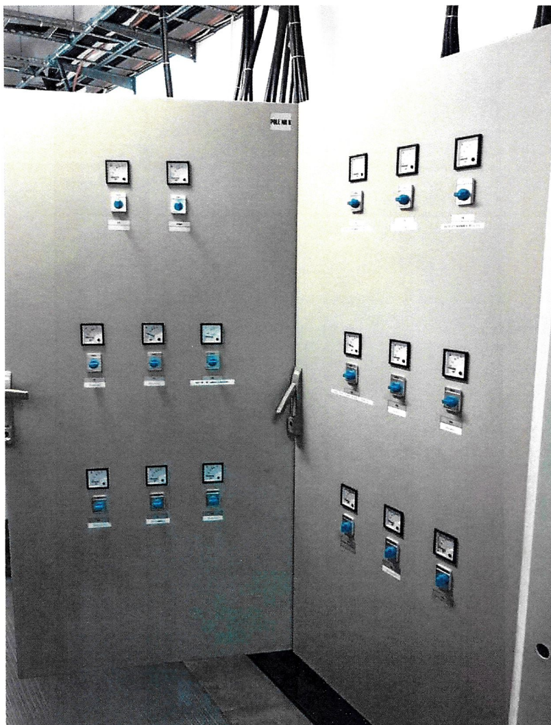
Widok rozdzielnicy R1-0 – fragment.
