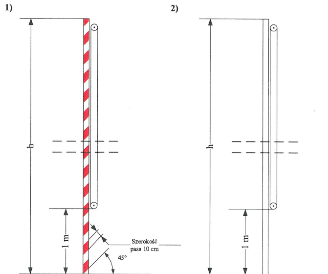
Rys. 1. Maszt flagowy: 1) biało-czerwony z określonymi parametrami, 2) biały z określonymi parametrami,
