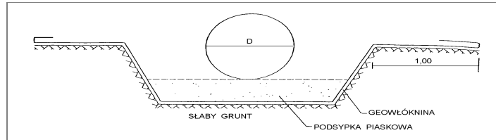
Rys. 5. Ułożenie rur przepustu na słabym gruncie
