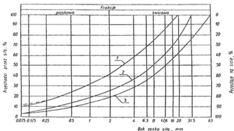
Rysunek 1. Pole dobrego uziarnienia kruszywa przeznaczonych na podbudowy wykonywane metodą stabilizacji mechanicznej
