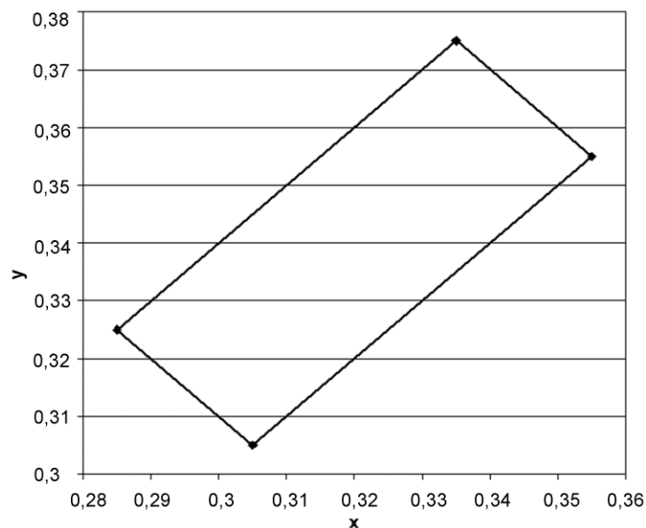
Rys. 1. Współrzędne chromatyczności x,y dla barwy białej oznakowania A
