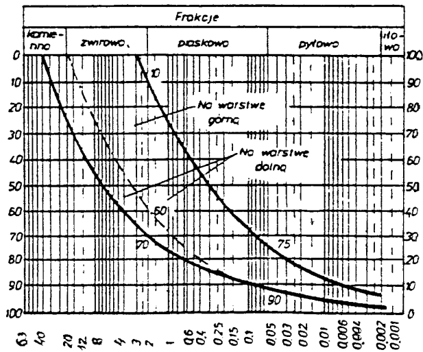
Rysunek 2. Obszar uziarnienia optymalnych mieszanek gliniasto-żwirowych
