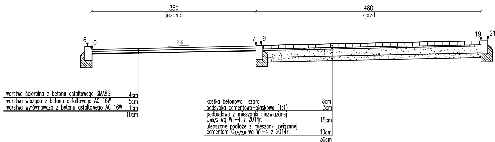
Przekrój II-II
