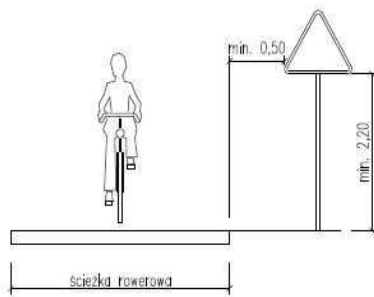
Rys. 3. Odległość znaków od krawędzi ciągu pieszo-rowerowego oraz wysokość umieszczania znaków.
