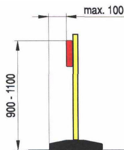
Rys. 8. Ustawienie zapory drogowej.
