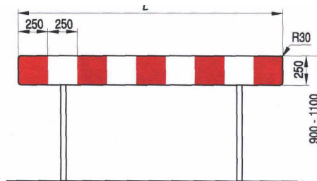
Rys. 3. Wzór zapory drogowej pojedynczej U-20a. L=750, 1250, 1720, 2250, 2750 mm.
