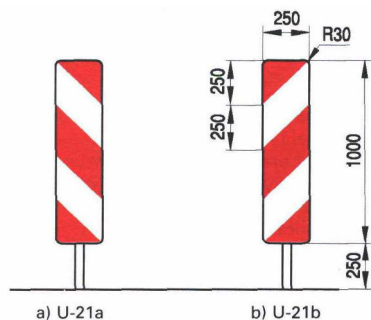
Rys. 7. Wzory tablic kierujących U-21a, U-21b
