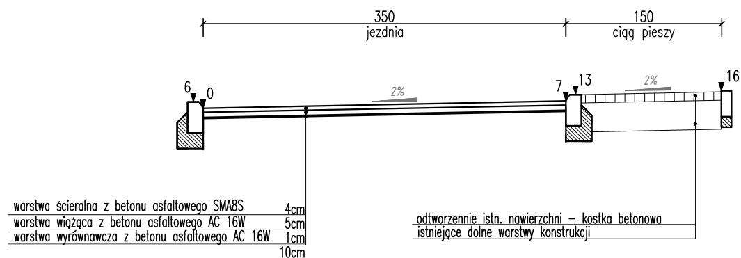
Przekrój I-I
