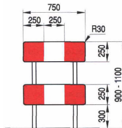
Rys. 4. Wzór zapory drogowej podwójnej U-20c
