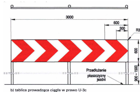
Rys. 6. Wzór tablicy prowadzącej U-3c
