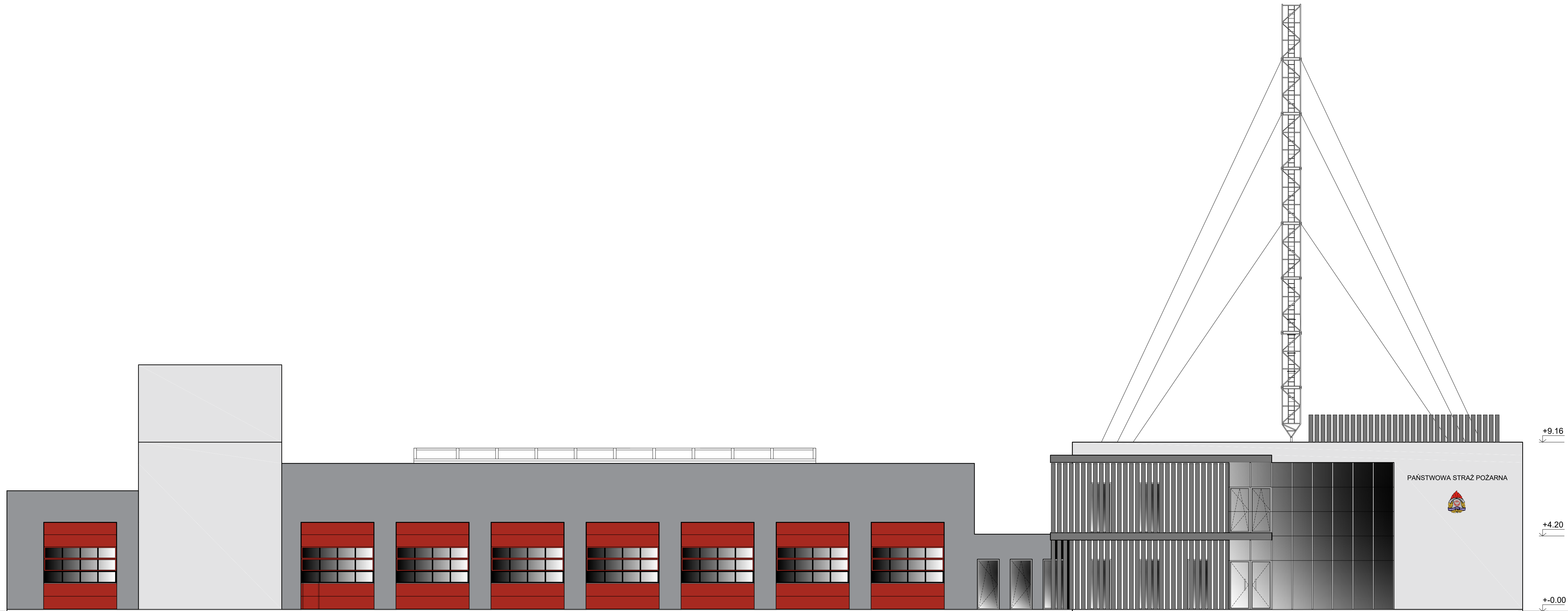
ELEWACJA ZACHODNIA
