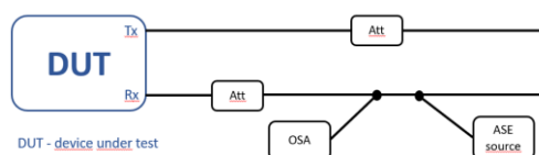
Rysunek 13.2. Schemat połączeń nr 2
