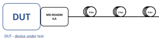
Rysunek 13.10. Schemat połączeń nr 10 – zasięg monitorowania włókien
