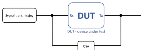
Rysunek 13.7. Schemat połączeń nr 7
