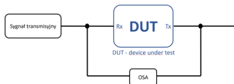
Rysunek 13.6. Schemat połączeń nr 6
