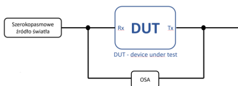
Rysunek 13.8. Schemat połączeń nr 8
