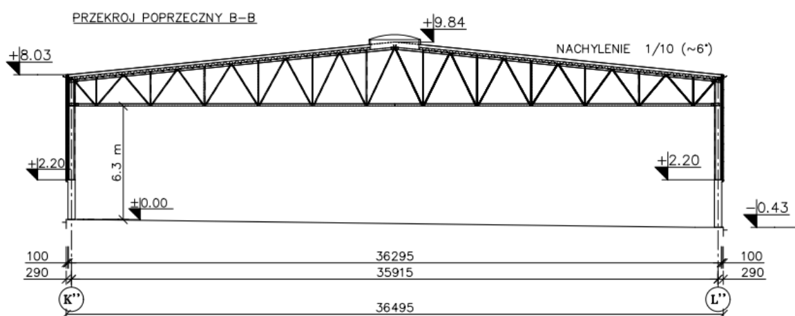
Rys.3 Przekrój poprzeczny obiektu 409C
